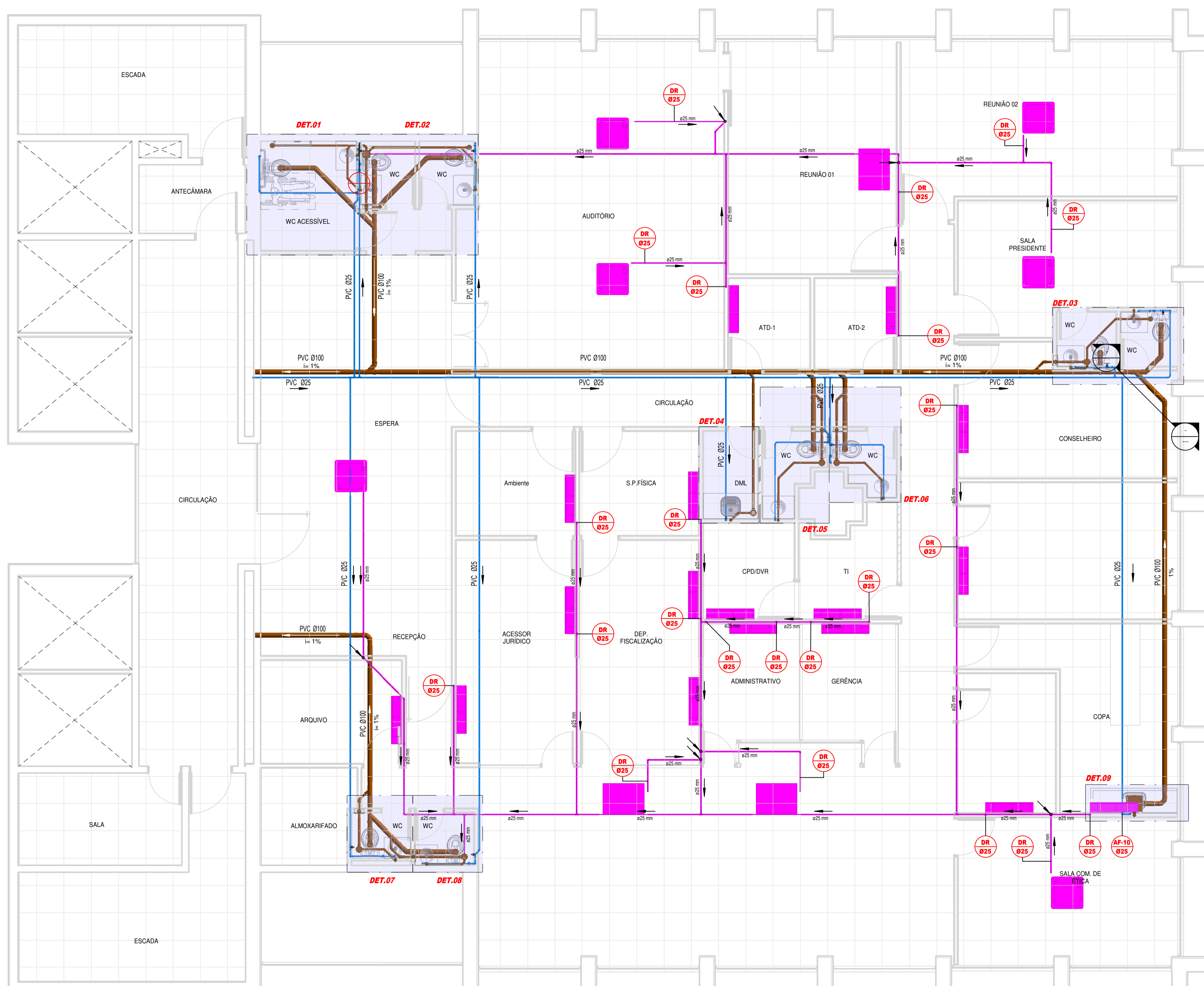
PLANTA BAIXA 1 : 50
